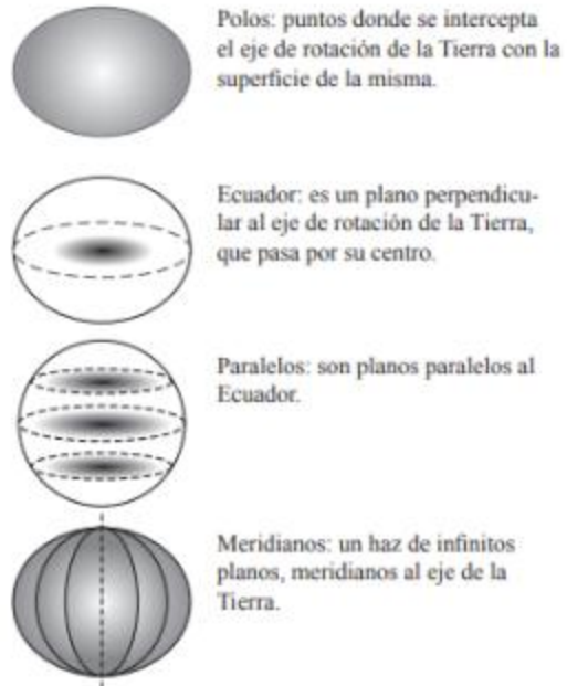
Figura 34. Componentes del sistema de coordenadas geográficas
